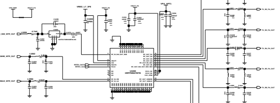
MMB (LTE 1/3/5/8/20, WCDMA 1/2/5/8, GSM LB/HB)
