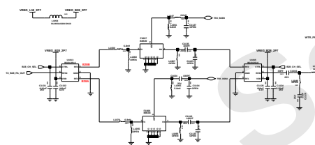
B28A/B28 DPX & B20/B28 PRx
